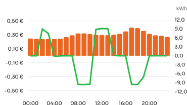
Thuisbatterij energie en uurprijzen
