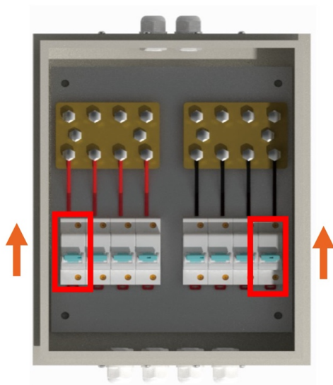
SET 6 L & SET 8 L: DC-4IN2OUT
